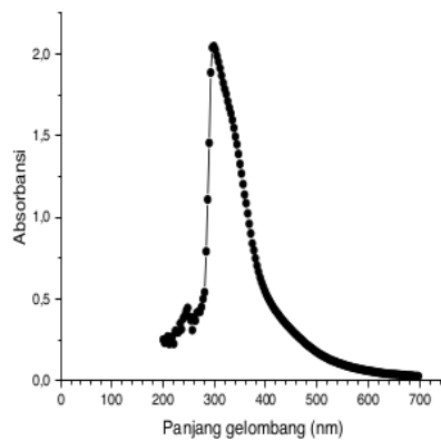
Gambar 3. Analisis panjang gelombang senyawa capsaicin
