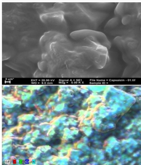
Gambar 4. Morfologi capsaicin menggunakan SEM-EDX
