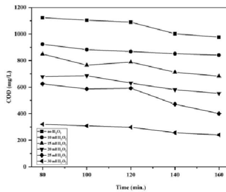
Gambar 2. Efek Perubahan COD terhadap waktu
