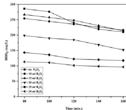
Gambar 3. Efek Perubahan BOD 5 terhadap waktu
