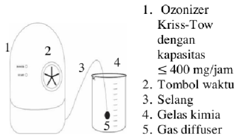
Gambar 1. Peralatan Proses Ozonasi
