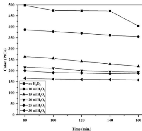
Gambar 4. Efek Perubahan Warna Terhadap Waktu
